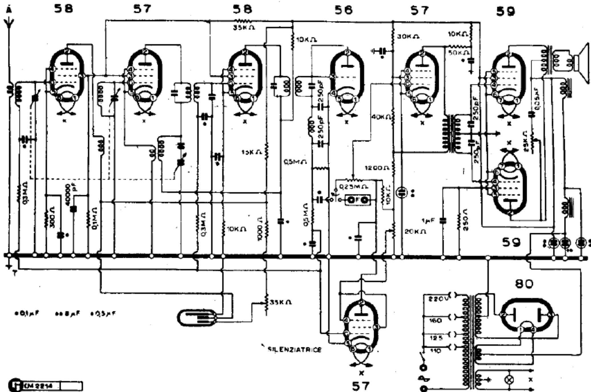
RADIO LAMBDA - MOD. « 329 »
